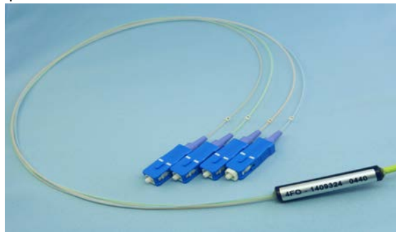
φ0.9mm分岐タイプ
